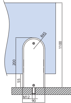
B-1020 Morsetto balastra Railing clamp Geländer Klemmhalter
